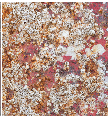
Bilderna visar hård påväxt på fartygsskrov. Den icke bevuxna sektionen på bilden i mitten har målats med Selektope-baserad färg.
