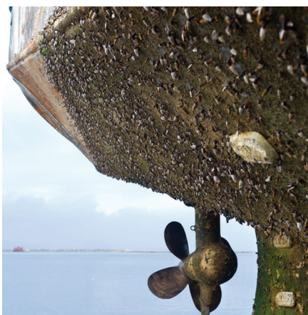
Bilderna visar hård påväxt på fartygsskrov. Den icke bevuxna sektionen på bilden i mitten har målats med Selektope-baserad färg.
